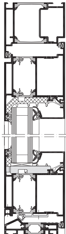
Schüco ADS 75 HD.II Schüco ADS 75 HD.II
